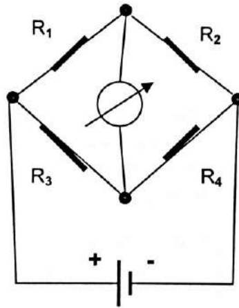
Figura 4 – Circuitos elétricos.
