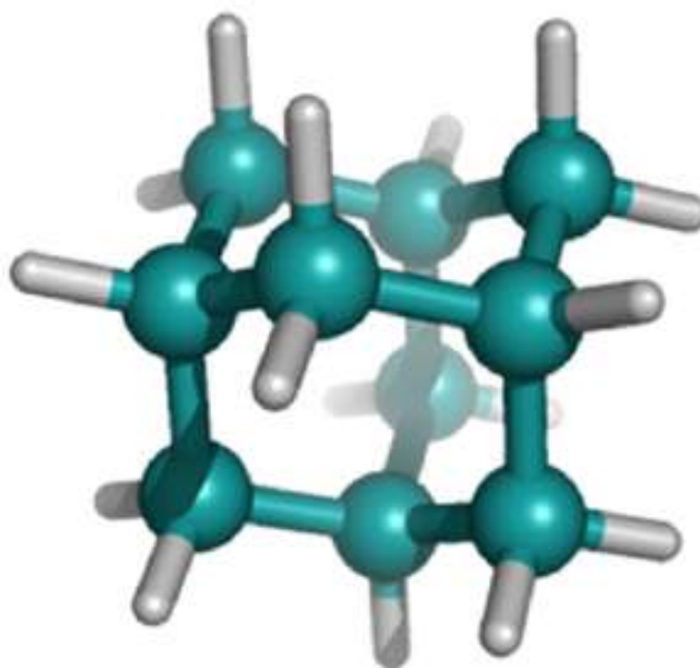
Figura 11 – Modelos químicos.
